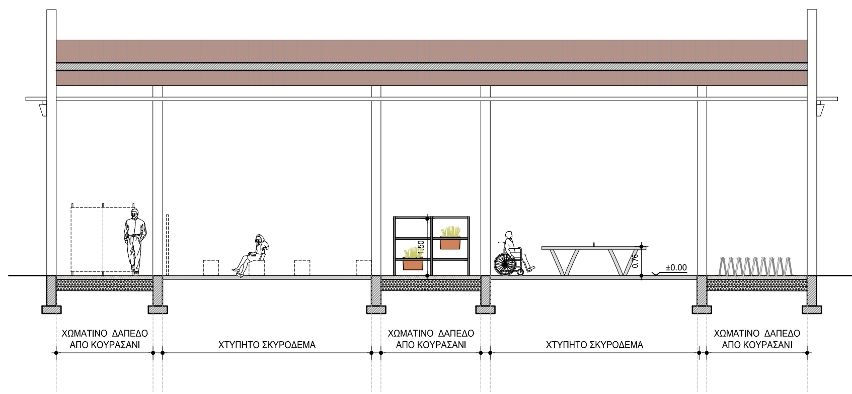
ΣΗΜΕΙΑΚΗ ΤΟΜΗ Α-Α
