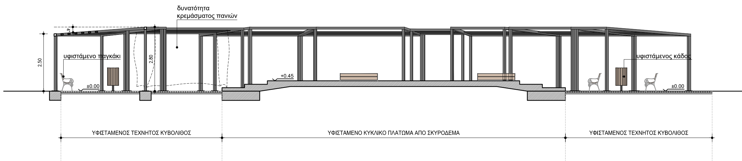
ΣΗΜΕΙΑΚΗ ΤΟΜΗ Β-Β
